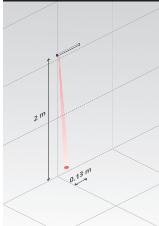
Diamètre du faisceau infrarouge 0,13 m @ 2 m
